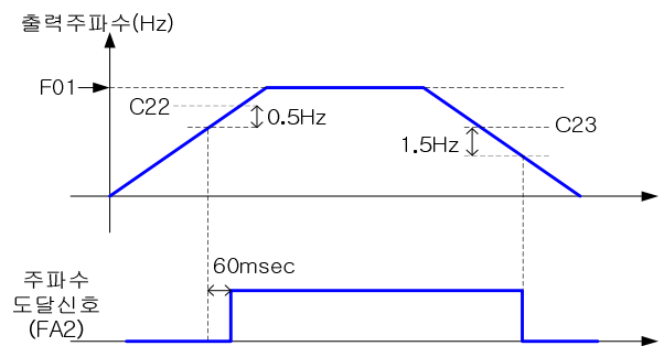
그림 5-58 주파수도달신호(FA2) 출력
