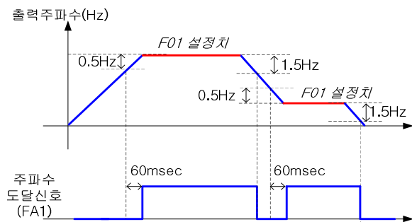
그림 5-57 주파수도달신호(FA1) 출력
