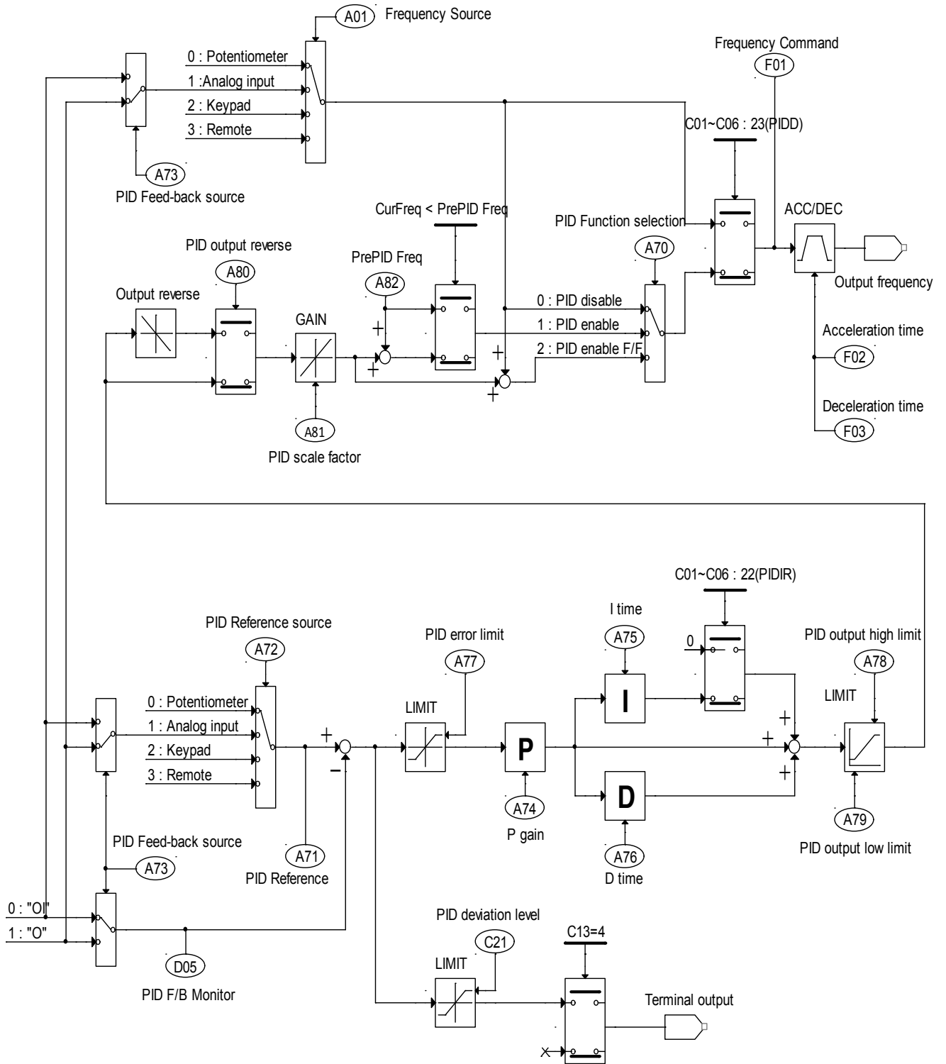
그림 5-16 PID 블럭도
